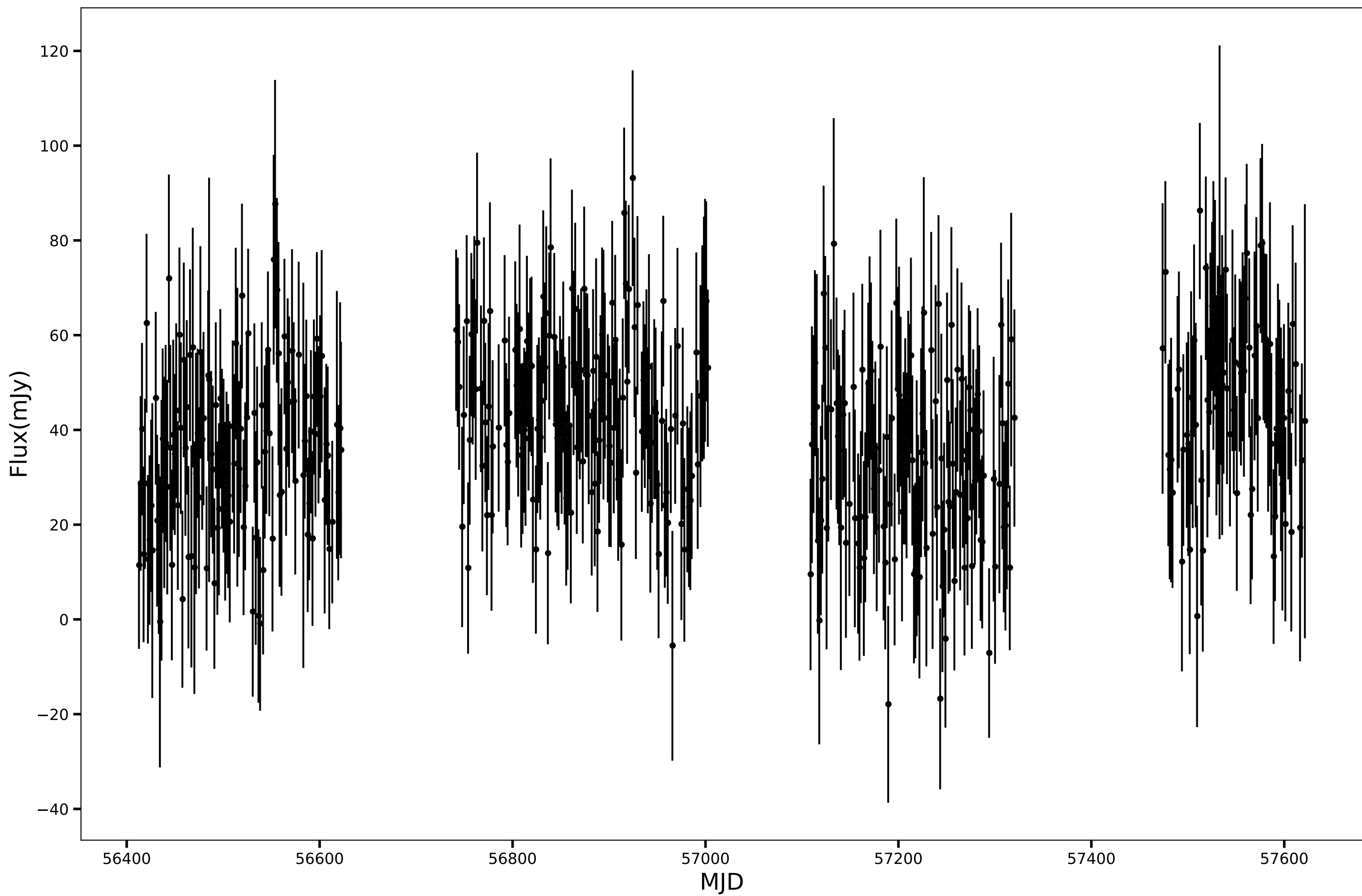
SPT-SJ221642-5637.5, RA=334.1768d, DEC=-56.6259d, mean_flux=39.26 (mJy), 90GHz
